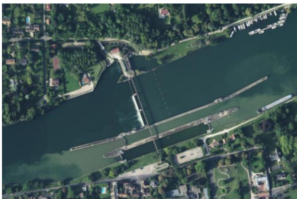
Barrage et écluse de la Cave
